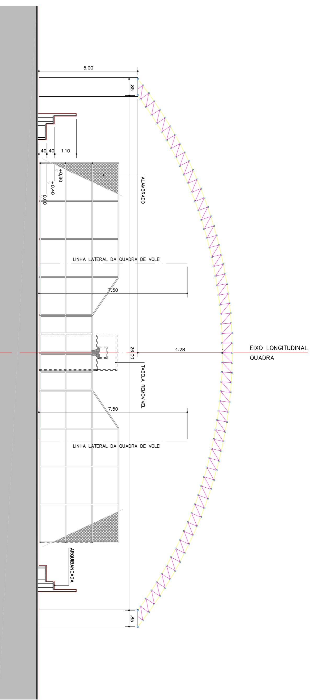
CORTE B-B ESC: 1:100
