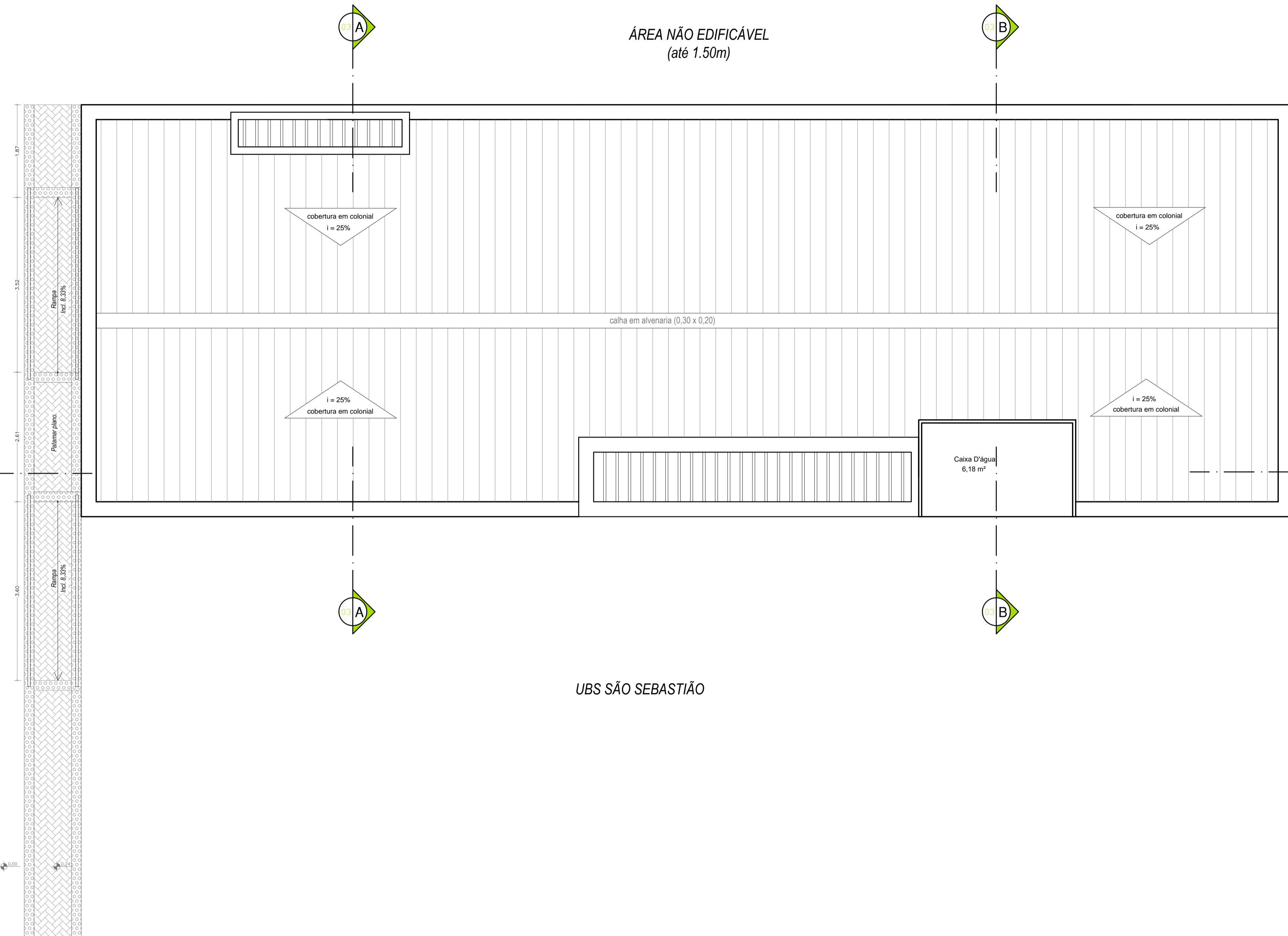
Planta Cobertura | Escala: 1:50
