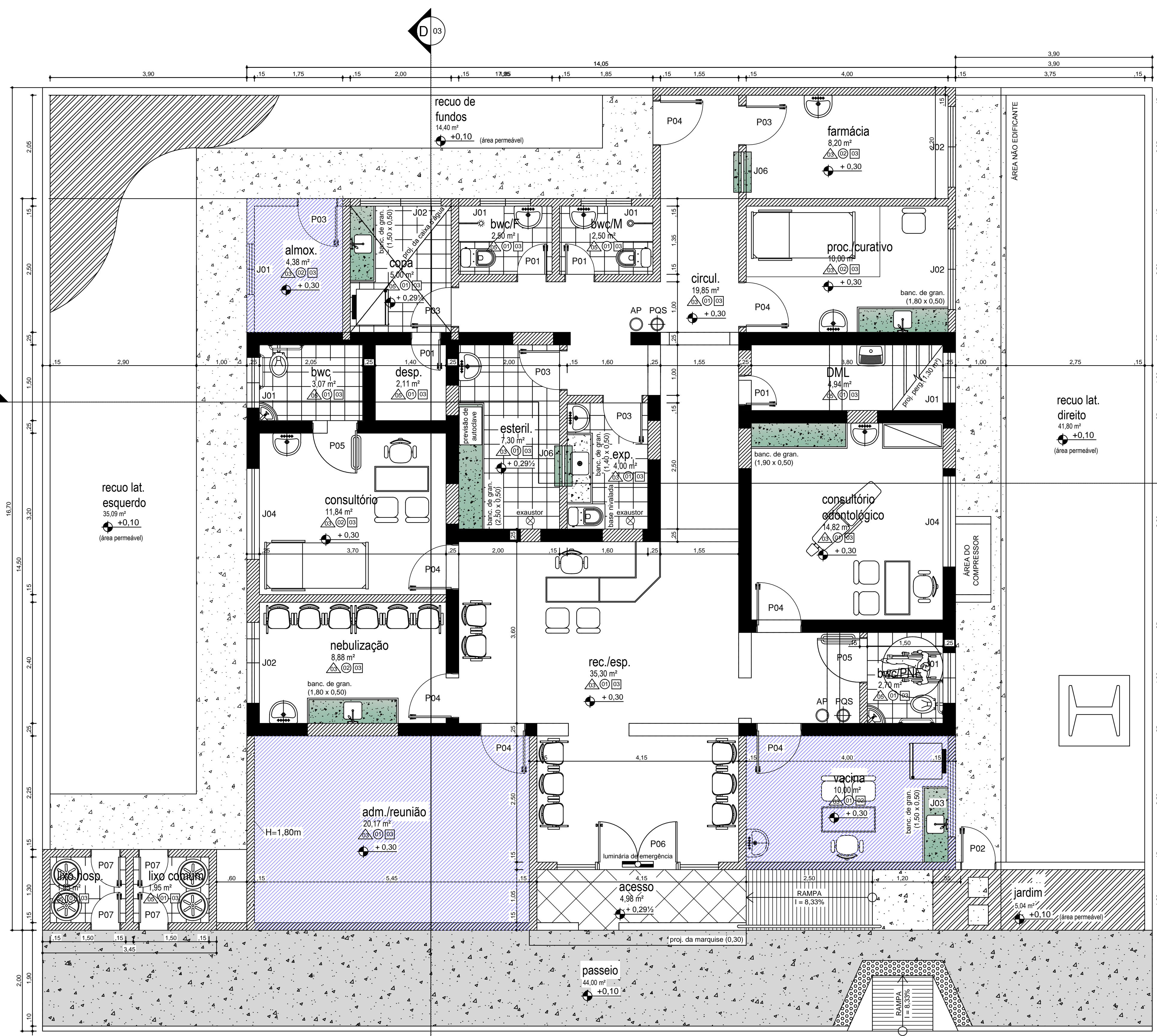
PLANTA BAIXA ESC. 1/50 ÁREA DE CONSTR. 217,47 m²
