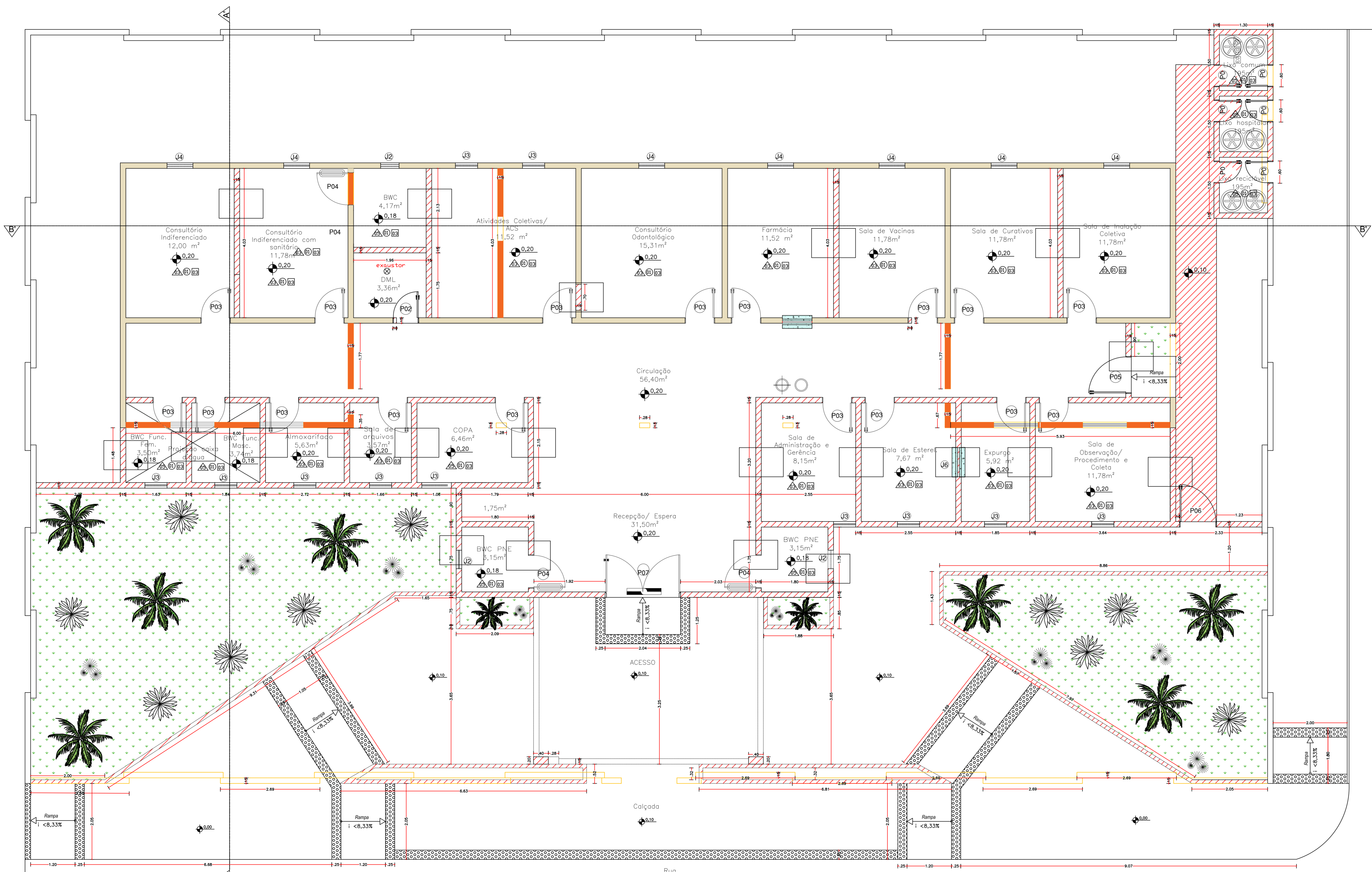
PLANTA DE REFORMA – Escala 1:50
