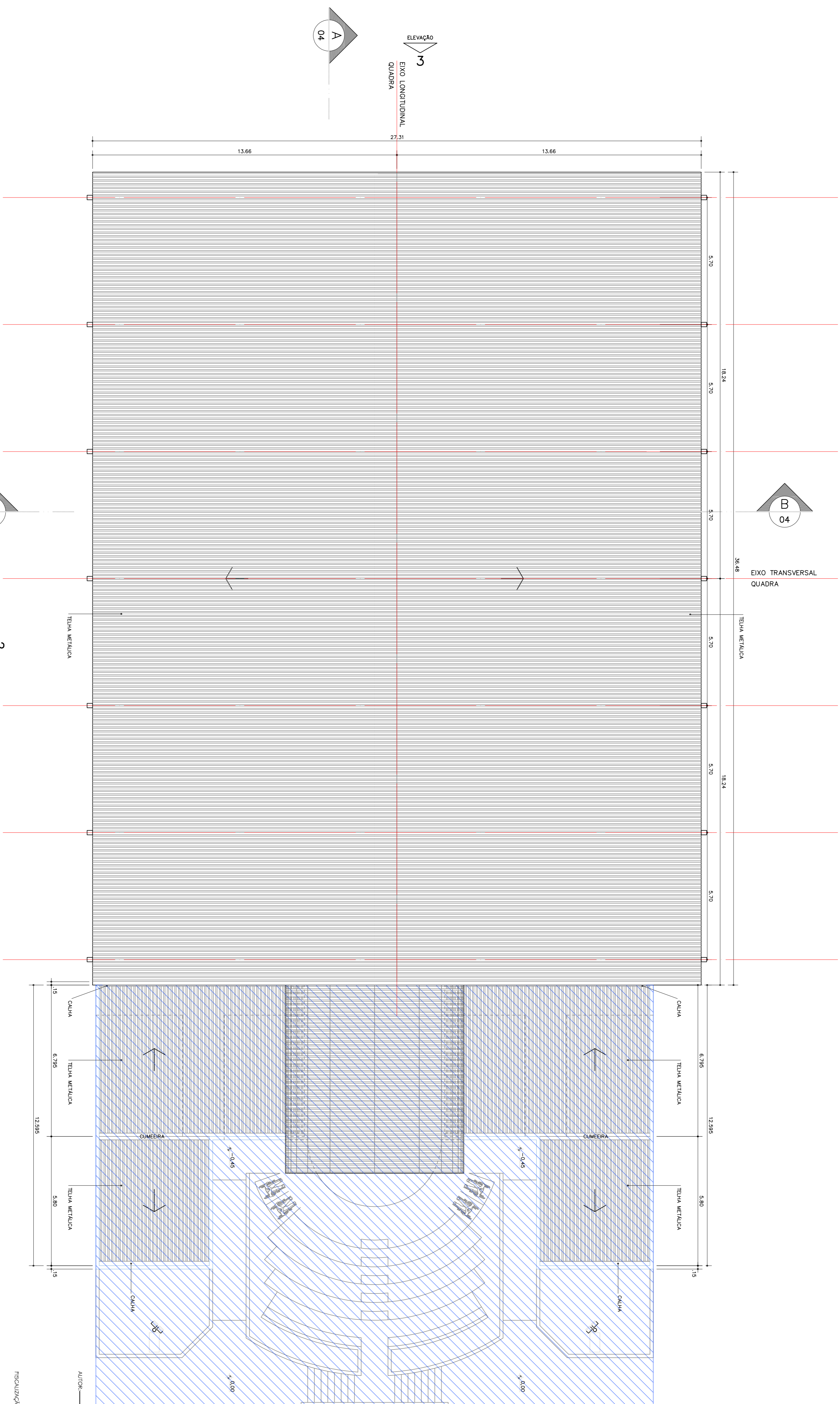
PLANTA DA COBERTURA Esc: 1:100
